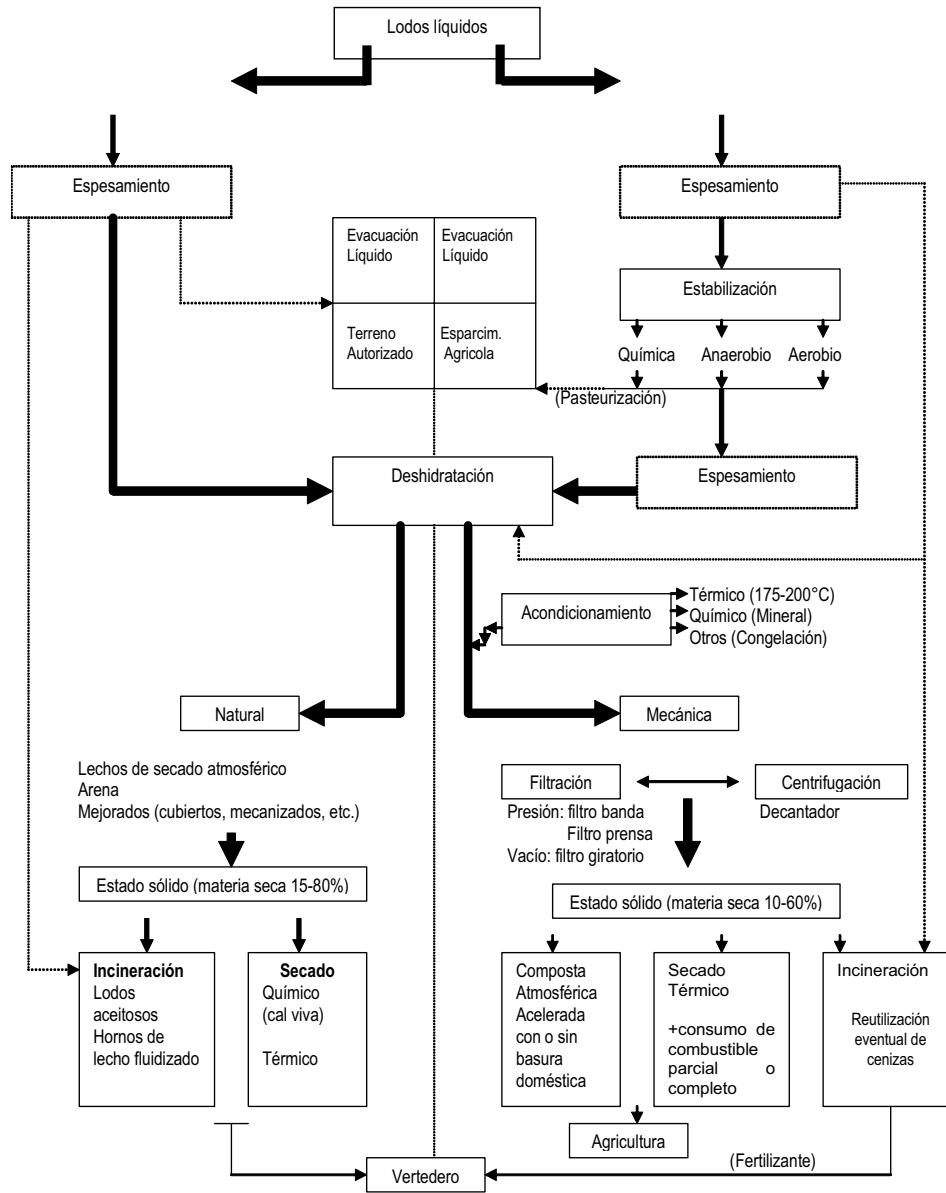
Figura 3. Líneas más comunes en el tratamiento de lodos (Dégremont, 1980).
