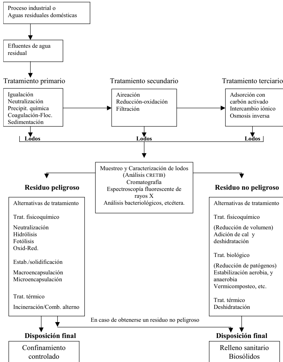
Figura 2. Alternativas planteadas para tratamiento y disposición de lodos.
