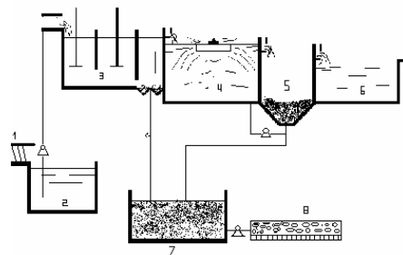
Figura 1. Arreglo de un sistema de lodos activados.
