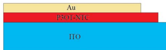
Estructura de la Celda Solar
